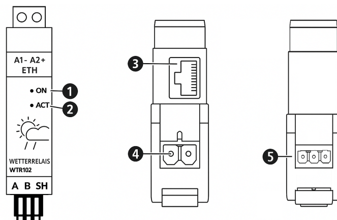
Abb. 1: Abbildung: Aufbau und Anschlüsse am Gerät.
