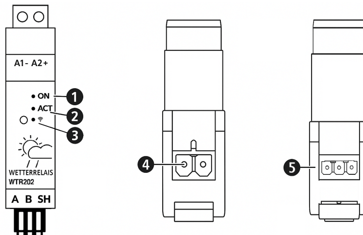
Abb. 1: Abbildung: Aufbau und Anschlüsse am Gerät.
